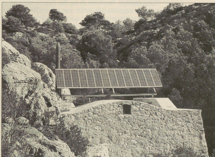
Instal·lació fotovoltaïca per a elevació d'aigua a sa Dragonera.
