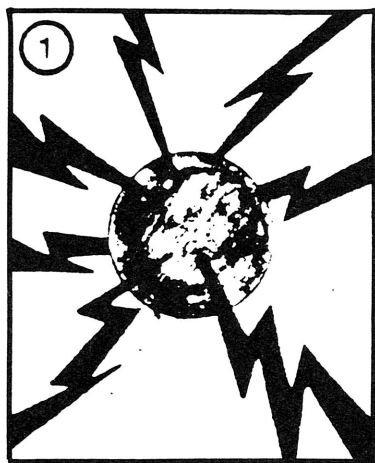
1. Impacte lluminós
