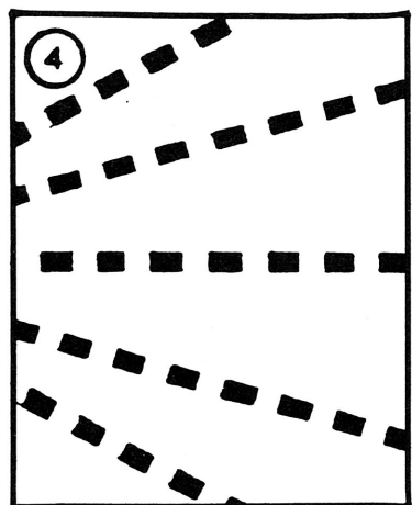
4. Radiacions
