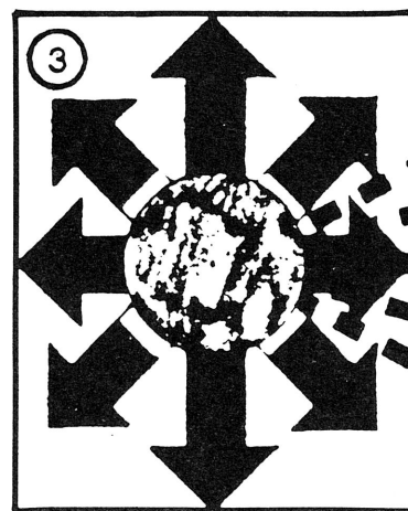
3. Esclafit atmosfèric
