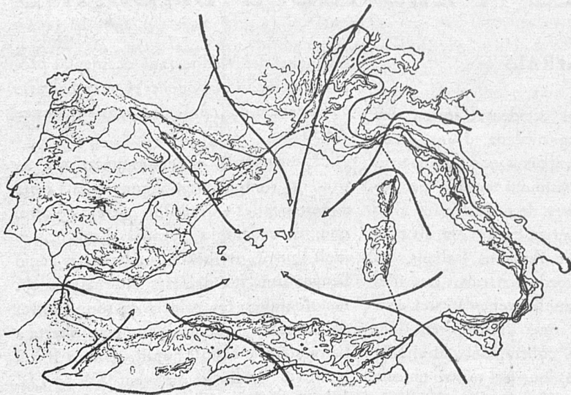
Línies d'isobari al Mediterrani Occidental. L'arxipèlag de les nostres Illes ocupa el centre de la cubeta, punt de concentració de totes les corrents, algunes d'origen molt llunyà.
