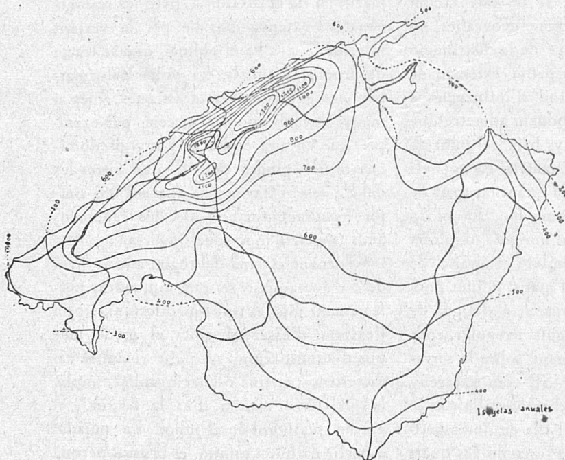
Distribució normal de la pluja sobre l'illa de Mallorca. Traços grossos: divisòries hidrogràfiques; traços fins: isoietes anuals normals o corbes d'una igual quantitat de pluja. Les xifres es poden interpretar indistintament com a milímetres d'altura, o bé com a litres per metre quadrat.
