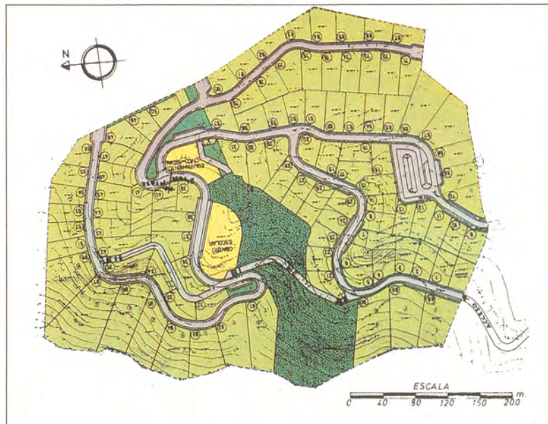
← Plànol de la parcel·lació de can Borràs (Andratx)
