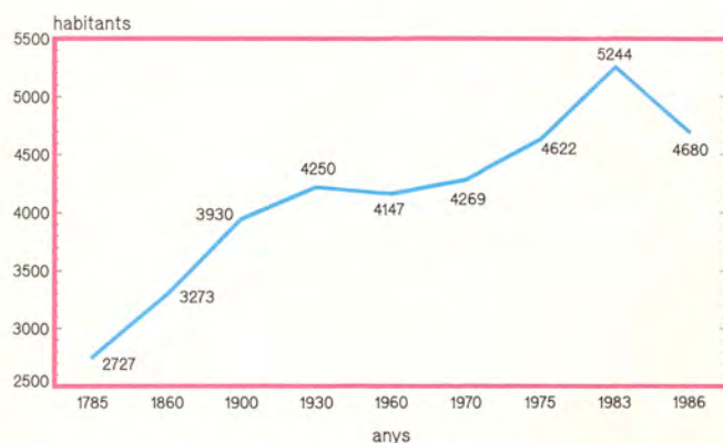
BINISSALEM Evolució de la població
