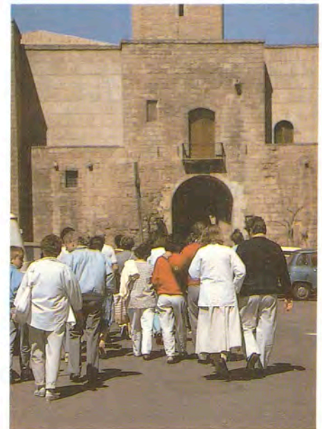
↑ El turisme augmenta la població de fet de les Illes
