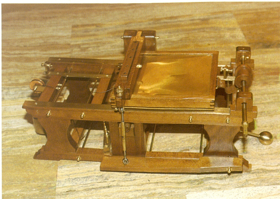
↓ Maqueta d'una antiga premsa plana d'impressió
