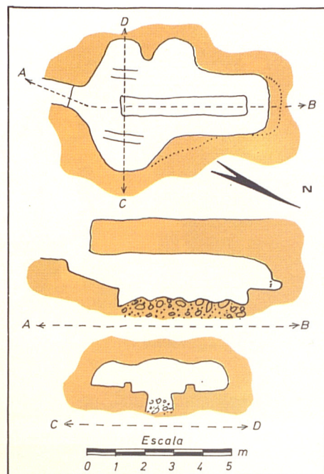
↑ Son Hereu (Llucmajor), plànol d'una de les coves prehistòriques de la pleta de sa Cova
