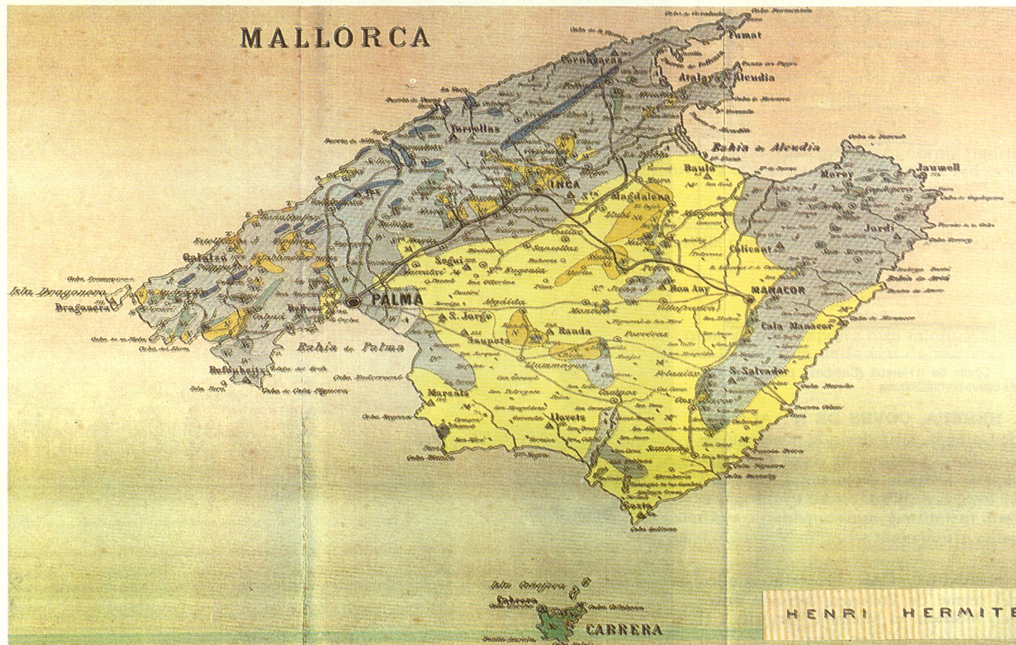
↓ Mapa geològic de Mallorca elaborat per Henri Hermite (AAM)
