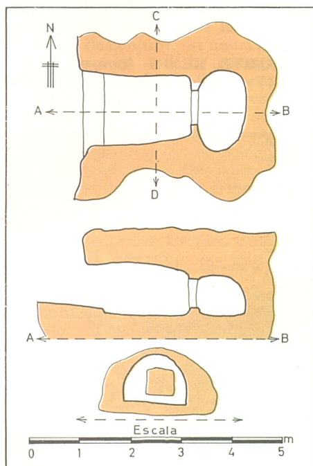
↑ Coves de n'Hereua (Campos), plànol d'una de les coves prehistòriques
