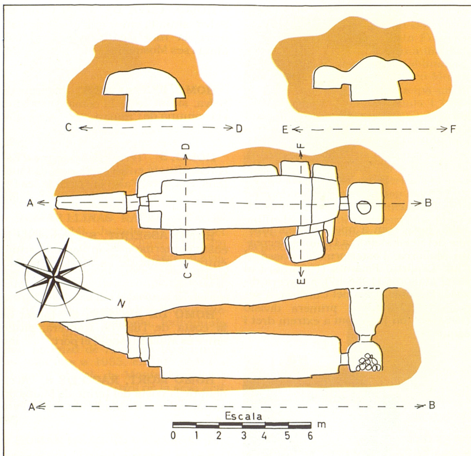
↑ Plànol de la cova de s'Homonet (Manacor)
