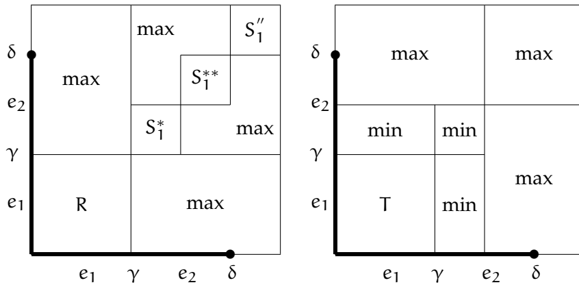
Figura 22. U_1 \in \mathcal{U}_{\cos, \max} (esquerra) distributiva sobre U_2 \in \mathcal{U}_{\min} (dreta), amb \gamma \leq e_2 < \delta .
