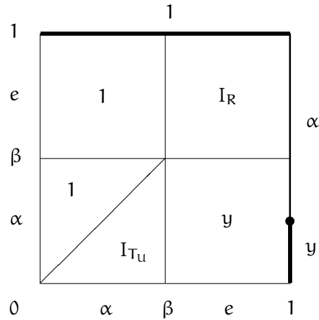
Figura 33. Estructura de I_U , amb U \in \mathcal{U}_{\cos, \min} .
