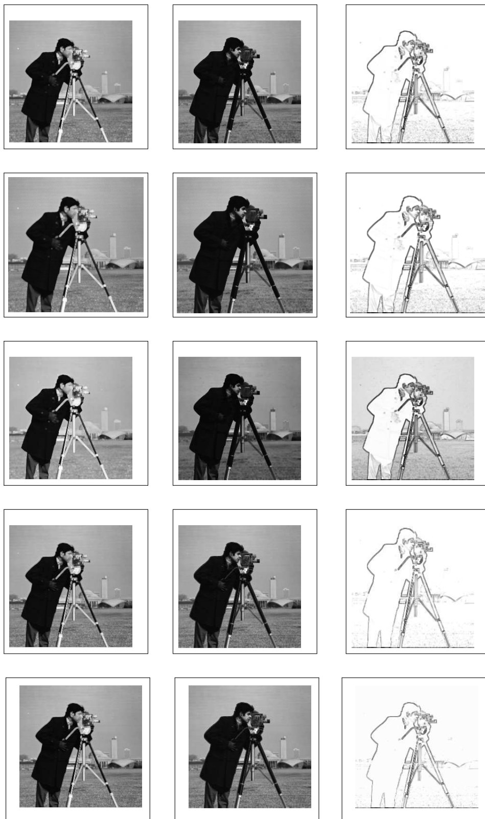
Figura 43. Dilatació borrosa, erosió borrosa i gradient borrós obtinguts emprant uninormes representables conjuntives amb generadors additius h(x) = \ln\left(\frac{x}{1-x}\right) , h_c(x) = \ln\left(\frac{-1}{\ln 2} \ln(1-x)\right) i h(x) = \frac{x-0.5}{x(1-x)} , la parella (T_L, I_T) i l'enfocament umbra.
