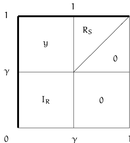
Figura 34. Estructura de I_U , amb U \in \mathcal{U}_{\cos, \max} .
