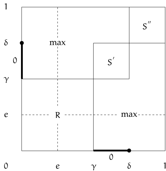
Figura 5. Estructura d'una uninorma de \mathcal{U}_{\cos, \max}
