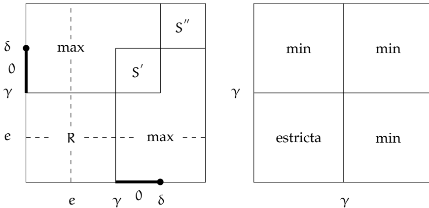
Figura 9. Uninorma U de \mathcal{U}_{\text{cos}, \text{max}} (esquerra) condicionalment distributiva sobre una t-norma contínua T (dreta).
