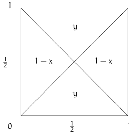
Figura 31. I_U amb U \equiv \langle N, \frac{1}{2} \rangle_{ide} i N(x) = 1 - x .
