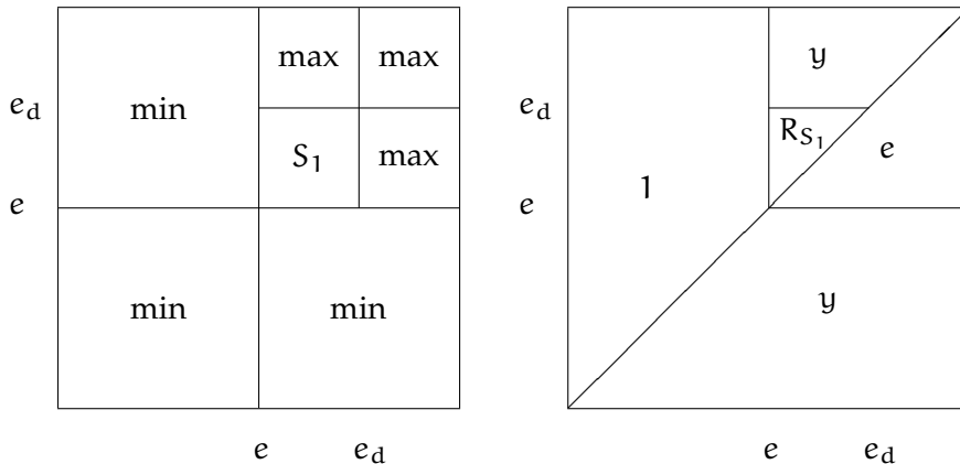
Figura 37. Una uninorma U (esquerra) de \mathcal{U}_{min} i la seva implicació residual I_U (dreta) tals que I_U, U_c i U_d satisfan (4.24), on U_c és idempotent de \mathcal{U}_{min} amb e_c = e i U_d \equiv \langle g_d, e_d \rangle_{ide} amb e_d > e i g_d(e) = 1 .
