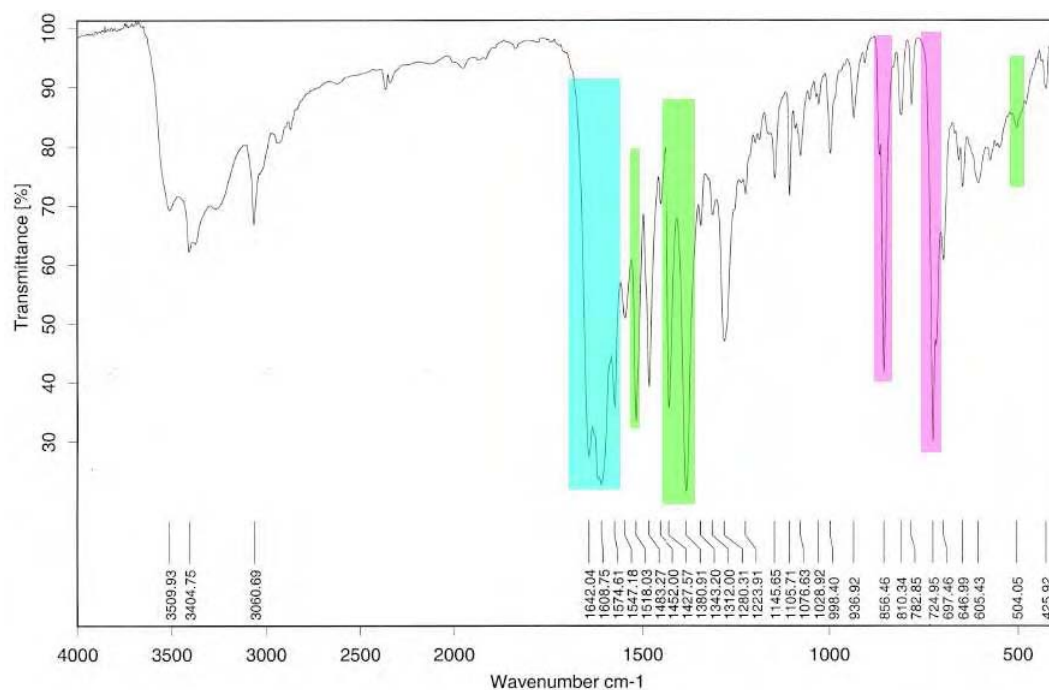
Figura 118. Espectre d'infraroig del complex [\text{Cu}(\text{I-hip})(\text{phen})_2]^+ (\text{I-hip}) \cdot 7\text{H}_2\text{O} [45]. S'han marcat en color rosa les bandes característiques de la 1,10-fenantrolina, en verd les corresponents al I-hip assignades per comparació amb els espectres dels binaris i en cel una zona en que s'hi inclouen les vibracions assignades a \nu(\text{C}=\text{O})_{\text{I-hip}} + \nu(\text{C}-\text{N})_{\text{I-hip}} + \nu(\text{COO})_{\text{I-hip}} + \nu(\text{C}-\text{N})_{\text{phen}} + \nu(\text{C}=\text{C})_{\text{phen}} .
