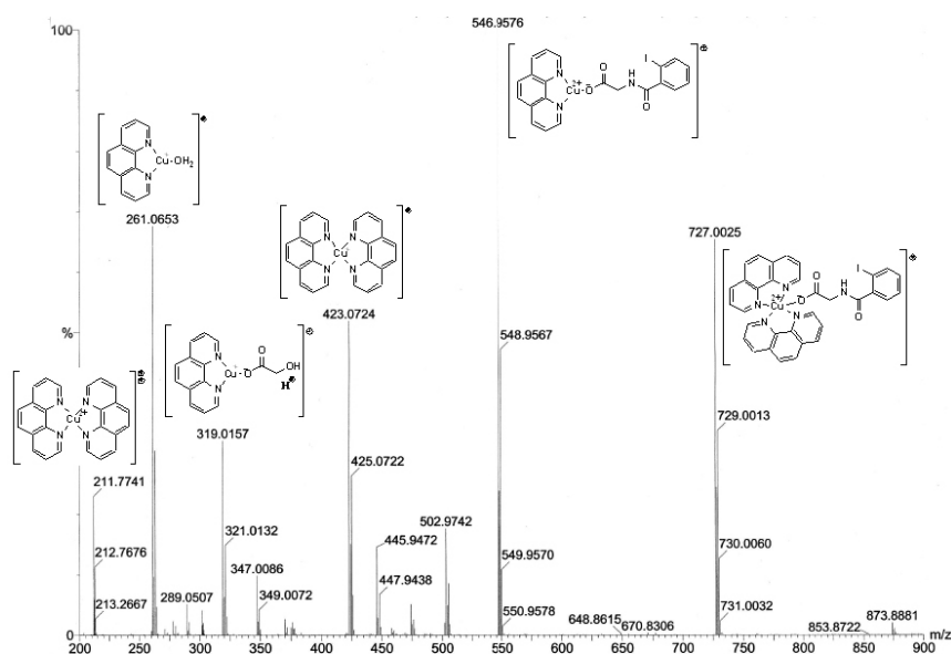
Figura 119. Espectre ESI-HRMS, en aigua, del compost [\text{Cu}(\text{I-hip})(\text{phen})_2]^+ (\text{I-hip}) \cdot 7\text{H}_2\text{O} [45] on s'observen els senyals corresponents a tots els composts detectats a l'inici de l'estudi cinètic (Figura 120).
