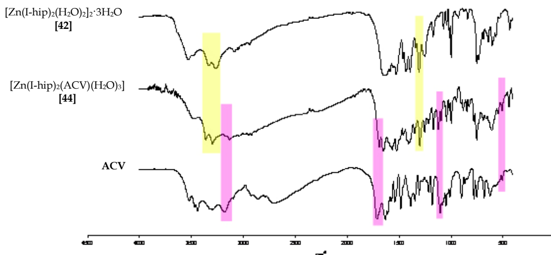
Figura 98. Representació dels espectres IR dels complexos binari [42] i ternari [44] de Zn(II) i de l'ACV (en rosa es marquen les vibracions provinents de l'aciclovir i en groc les corresponents al binari de I-hip)
