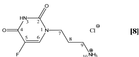
Figura 33. Fórmula i numeració del producte d'eliminació de l'ftalimida, el clorhidrat de N 1 -(3-aminopropil)-5-fluorouracil [8].
