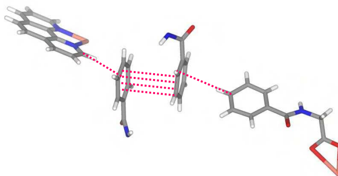
Figura 108. Clúster d'interaccions C-H···π···π···H-C al complex [46].
