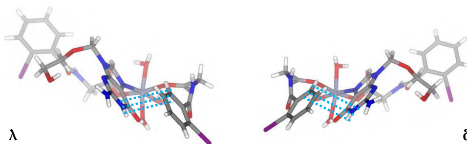
Figura 94. Representació dels dos enantiòmers presents al cristall del complex de Zn(II) amb la interacció per apilament indicada amb línies discontinües (-----).
