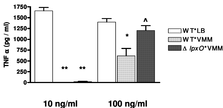
Figura 49: Cuantificación, mediante ELISA, de la secreción de TNF \alpha en MH-S tras ser estimulados con dos concentraciones diferentes de los lípidos A obtenidos. * indica una diferencia estadísticamente significativa (*P < 0.01, **P < 0.001, análisis de varianza de una cola ANOVA) con respecto al lípido WT*LB. (^P < 0.05, análisis de varianza de una cola ANOVA, con respecto al lípido WT*VMM).
