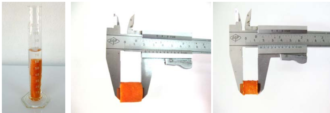
Figura 3.11. Medida del volumen y longitud de las muestras durante el secado por aire caliente de cilindros de zanahoria.
