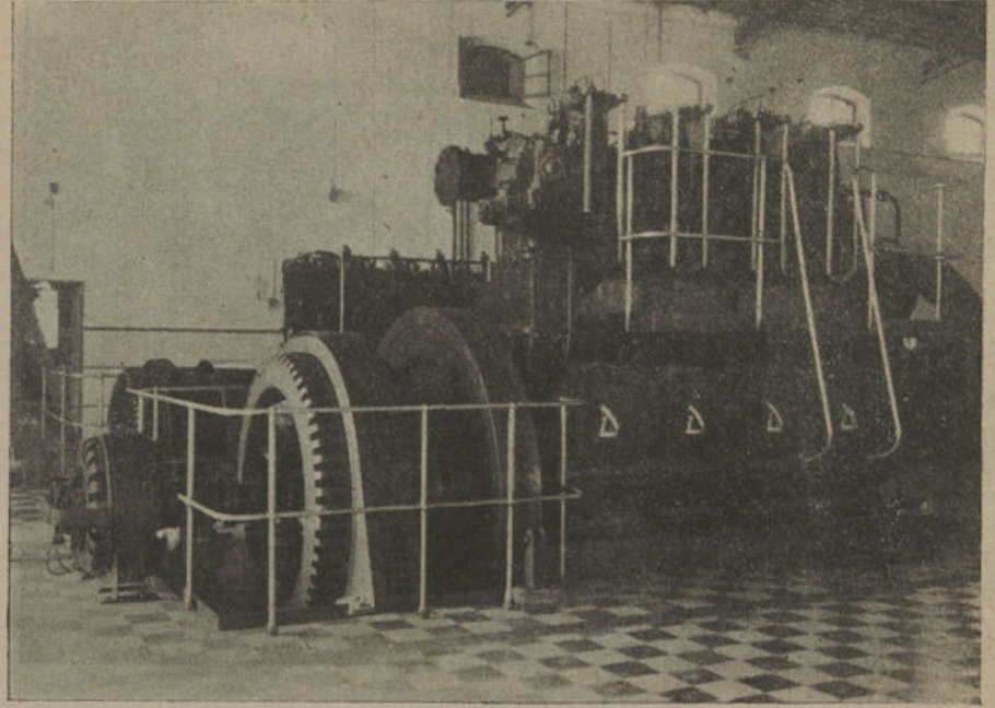
Motor Diesel, de 400 H. P., que acaba de ser instalado
