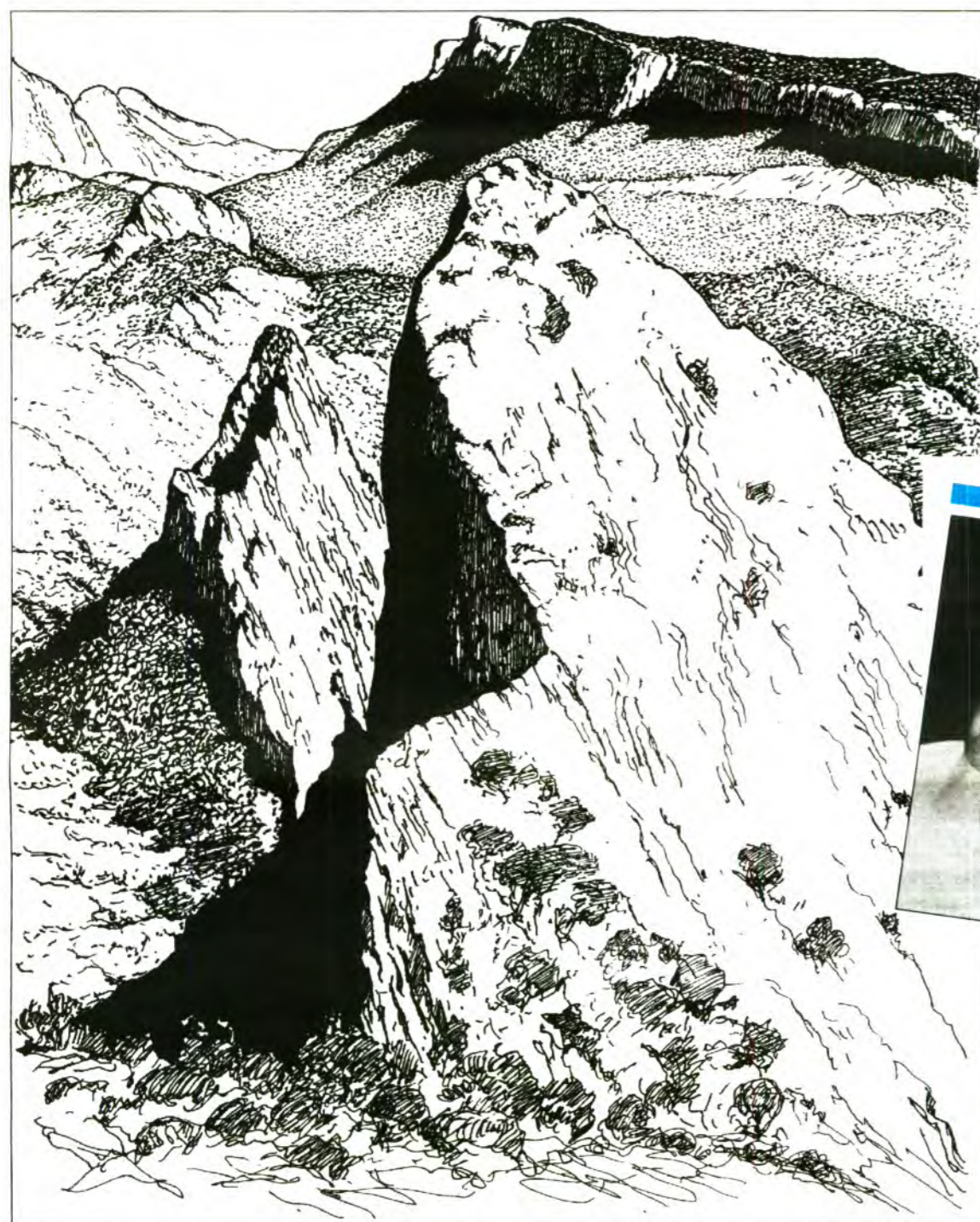
Aquest dibuix de Guillem Colom mostra el costat esquerre de la carretera Palma-Sóller, entre Can Penaso i Binifarani, on hi ha aquestes calisses líssiques. Al fons veim la sèrie tectònica de la Comuna de Bunyola i en darrer terme la iniciació de la vall sinclinal d'Orient.
