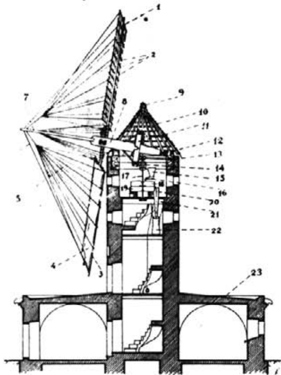
1. Tall vertical d'un MOLÍ DE VENT de les illes Balears, amb la nomenclatura de les seves peces principals:
