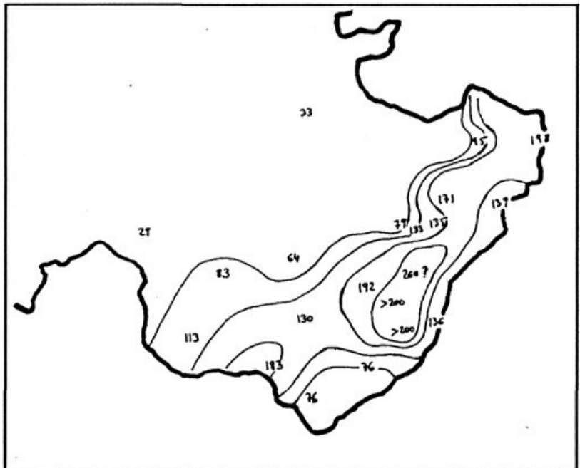
Fig. 3.- Mapa pluviomètric provisional del Llevant de Mallorca per als dies 5 a 6 de Setembre de 1989. Estan dibuixades les isoietes de 80, 120, 160 i 200 l/m 2 . (dades del Centre Meteorològic).
