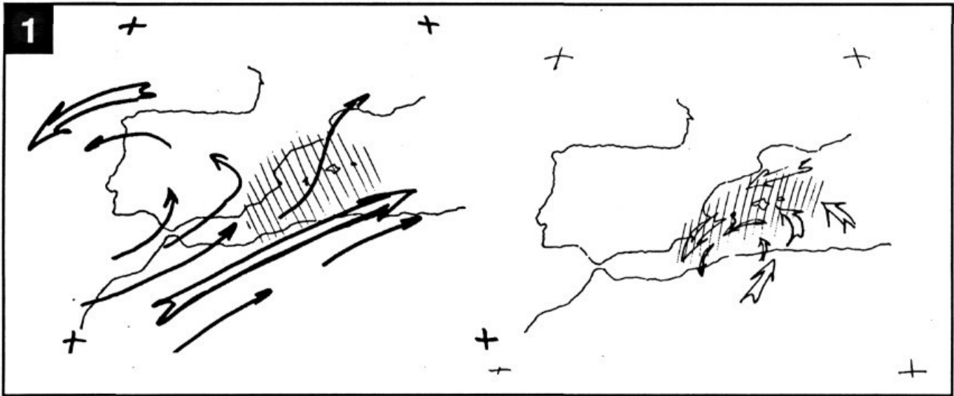
Fig. 1.- Esquema de la circulació atmosfèrica en nivells alts (esquerra) i nivells baixos (dreta). La zona rallada té possibilitat de formació de nuclis tempestuosos.
