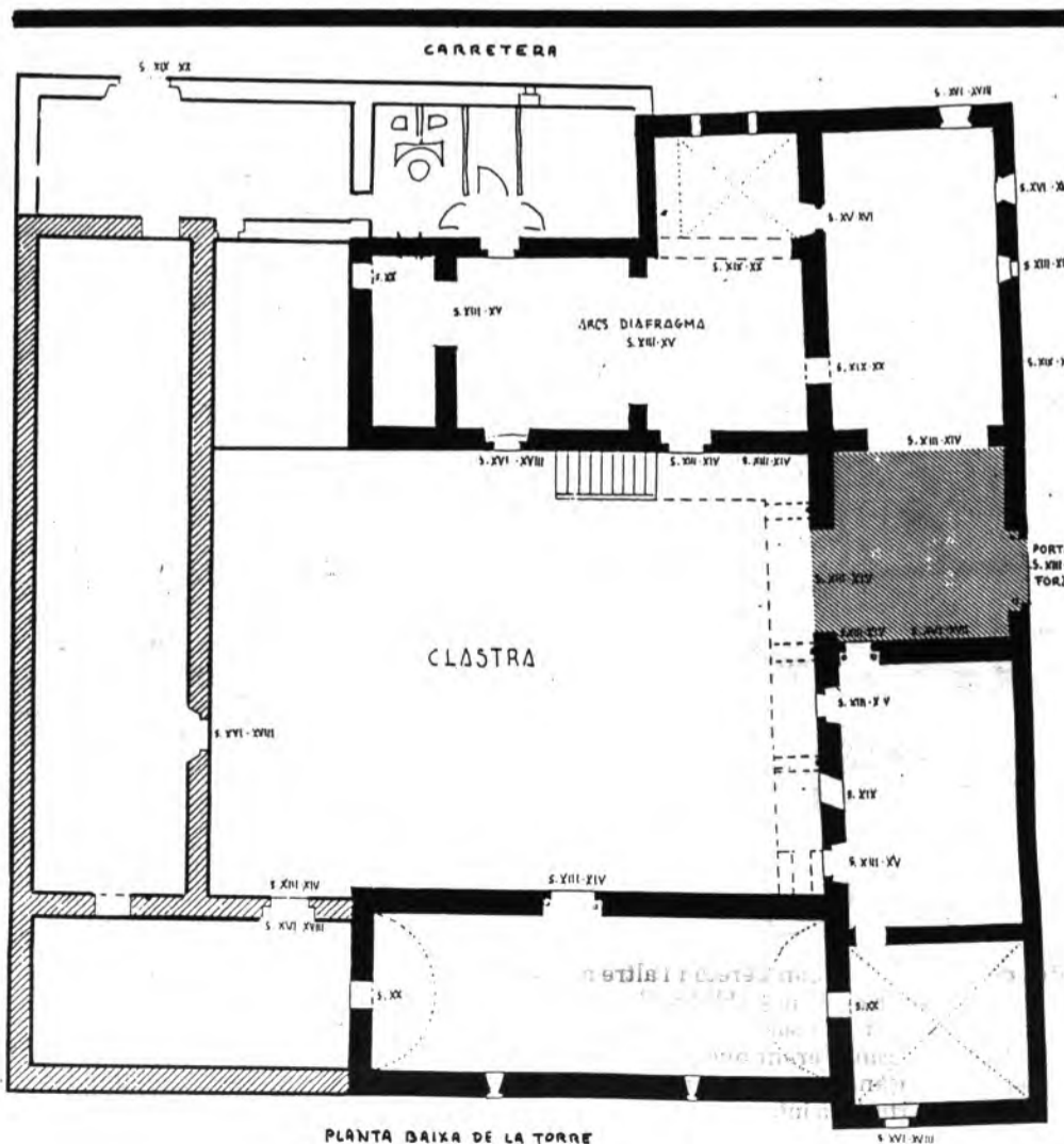
PLANTA BAIXA DE LA TORRE
