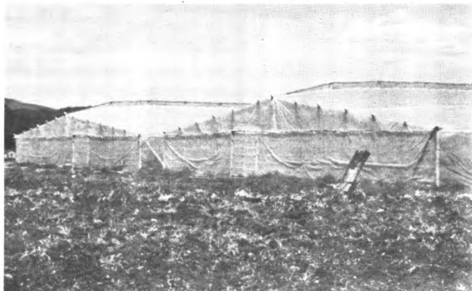
Panorámica de invernaderos de vigas pretensadas.
