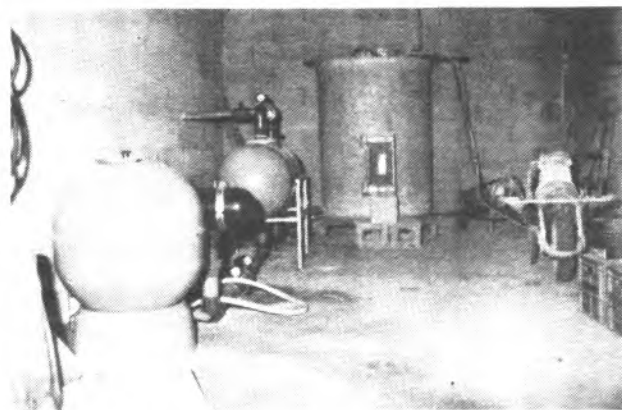
Equipo de alimentación. En primer plano abonadora; en segundo plano equipo de filtrado y al fondo red de sulcatados y desinfectados.
