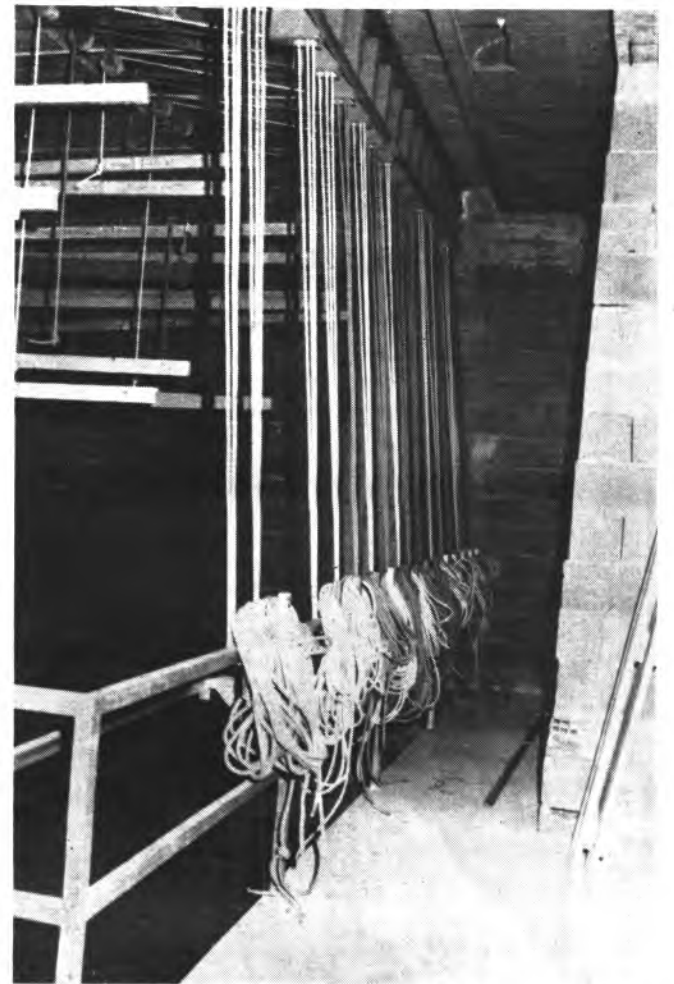
-El pasillo-balcón, con los cordajes dispuestos. Las cuarenta y cinco cuerdas, tensadas y a punto de poder manejarse.
