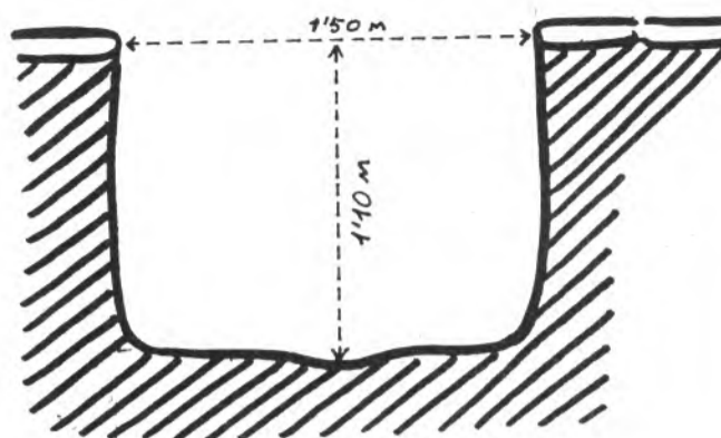
Corte ideal de la pileta o depósito.
