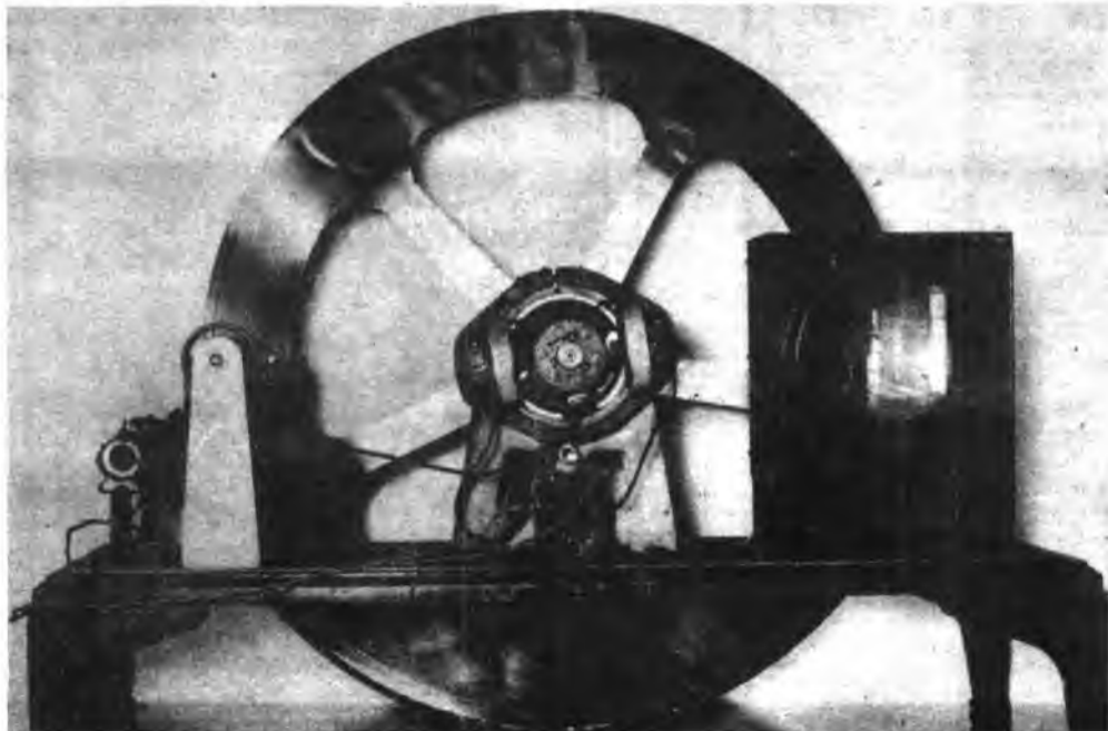
Un "televisor" del año 1929, cuyo funcionamiento se basaba en el llamado "disco de Nipkov", relegado muchos años a simple experimento escolar.
