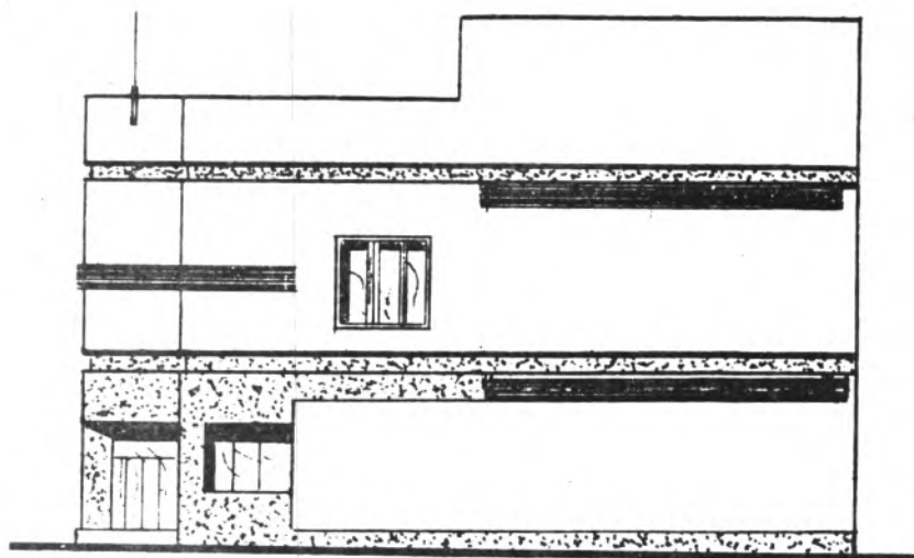
ALZADO CALLE SAN VICENTE
