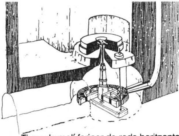
Tipus de molí fariner de roda horitzontal
