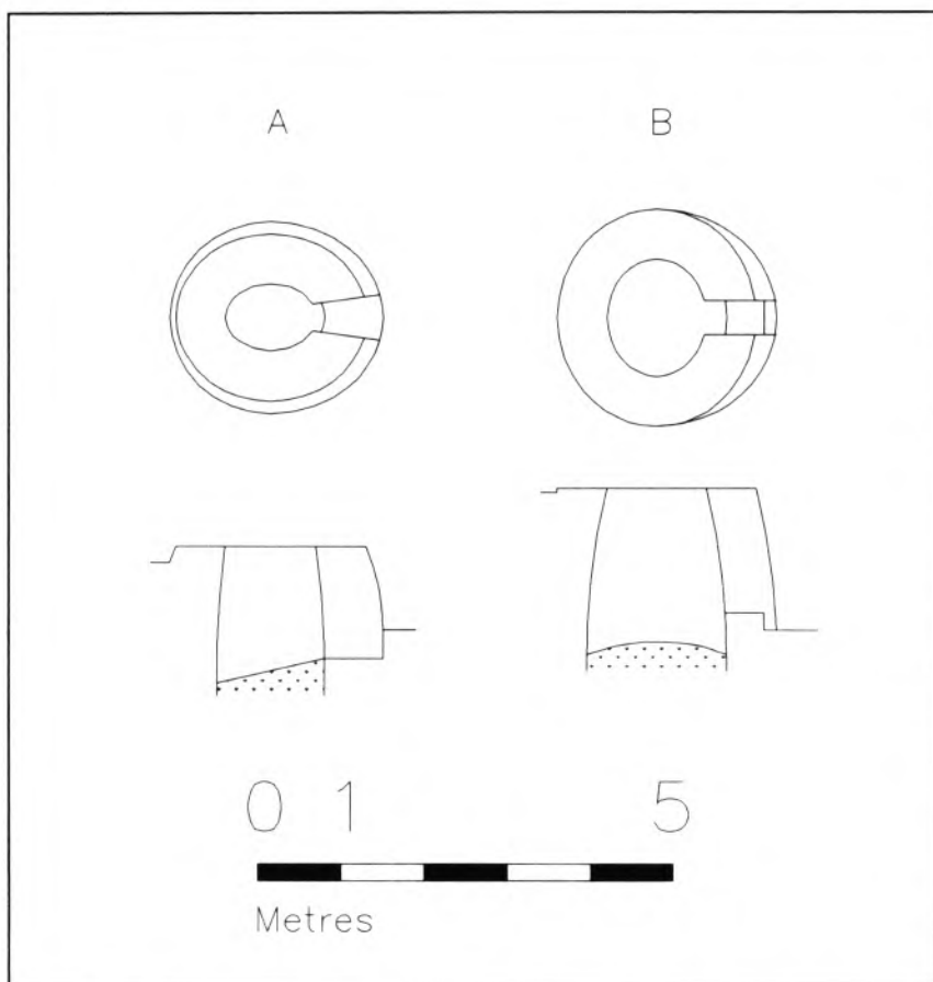
Figura 1. Planta i alçat de dos forns de guix valldemossins: A. Forn de guix des Guix (s'Estaca). Es troba molt prop de la mar, davallant-hi per un camí de carro, entre la rota des Figueral i la platja des Guix. B. Forn de guix des Guixet. Es troba a la falda de sa Comuna, un poc més avall que la casa de neu de Cartoixa. Just devora, hi ha una antiga pedrera de guix.
