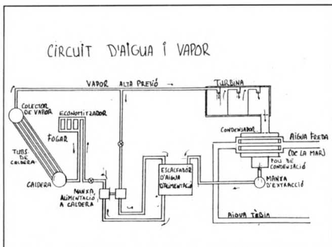
Dibuix 6 El vapor produït dins la caldera flueix a la turbina; dins aquesta el vapor passa pels diferents esglaons o seccions on perd pressió dins cada un d'ells, cedint la seva força a les pales de la turbina. Quan surt el vapor pel forat d'escampament del fons de la turbina passa al condensador; allà es condensa (produint un buït), quan es posa en contacte amb uns tubs pels quals circula aigua freda (1). El vapor condensat, recollit dins un pou, és succionat per la manxa d'extracció i el duu a l'escalfador de l'aigua d'alimentació, on es recalenteix de bell nou, essent posteriorment bombejat a la caldera, passant abans per l'economitzador situat dins el focar.
