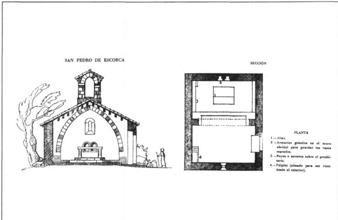
Secció de l'església de Sant Pere d'Escorca, contemporània de l'oratori de Sant Joan, del segle XIII (dibuix de G. Alomar).
