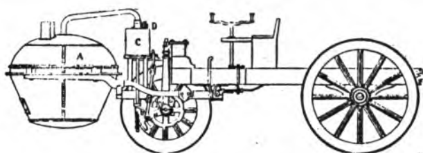
Auto-mòvil a vapor de Cugnot (1.770)
