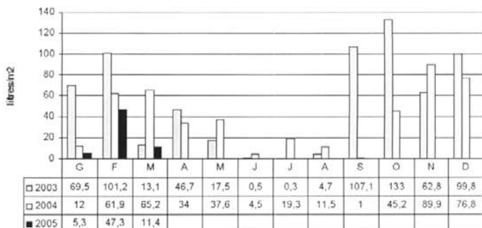
Pluviometria Comparativa
