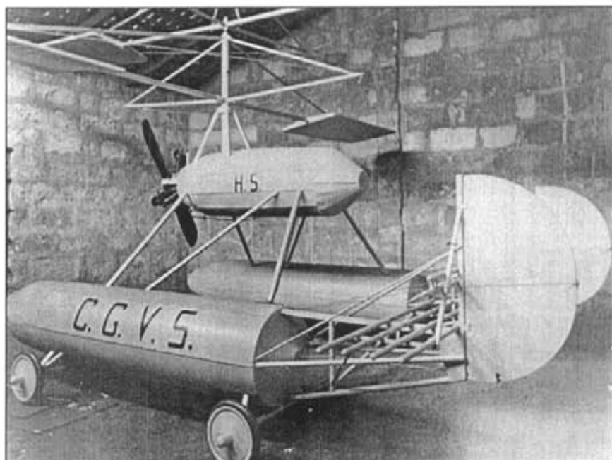
Magnífica vista lateral del COMETAGIROAVIÓ SASTRE (o hidroavió Sastre, com volia, també l'inventor) dins "l'hangar" de Son Gall. Es poden veure els dos flotadors o aerons descansant sobre quatre rodes amb una coberta de goma plena. A sobre de l'eix vertical superior hi ha acoplats dos parells de pales que fan la funció d'hèlices de sustentació. L'hèlice de davant de tot és la de propulsió, per a l'avançament horitzontal.
