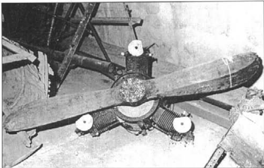
Motor d'aviació de tres pistons en estrella de 25 HP comprat a París a la casa de motors d'aviació Anzani. Va costar 13.000 francs.
