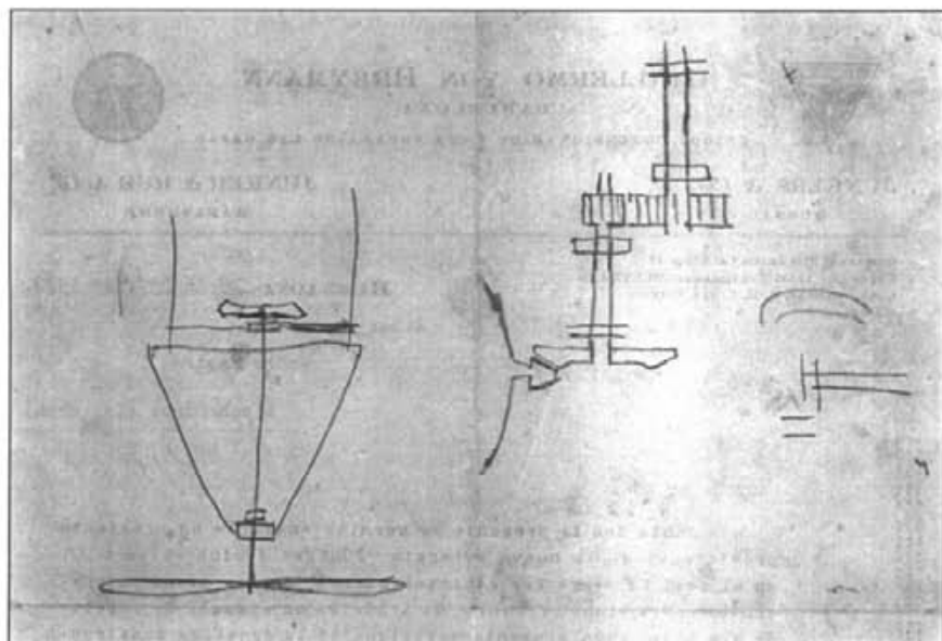
Croquis de mecanismes transmissors de forces
