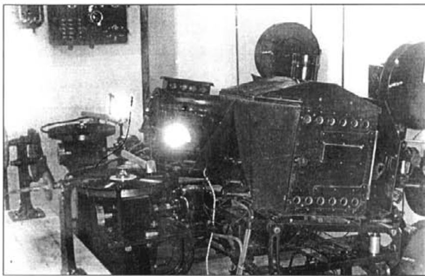
Maquinària de projecció del Recreatiu de Lluçmajor, amb el primitiu sistema sonor Vitaphone de tocadiscs (Recreatiu, Lluçmajor)
