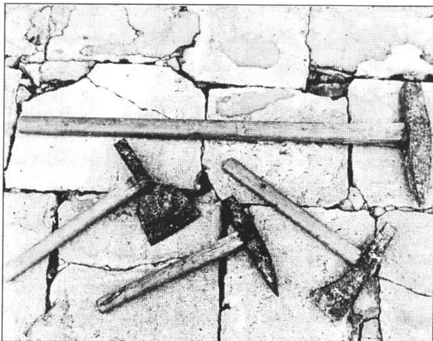
Picó gros, martell de tall de marès, martell de tall de pedra viva i martell amb punta.
