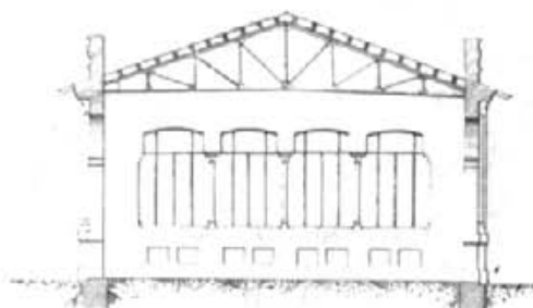
SECCIÓ AB.
