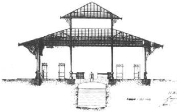
Façana i secció del projecte per un mercat municipal realitzat al 1909 per l'Arquitecte Gaspar Bennassar.
