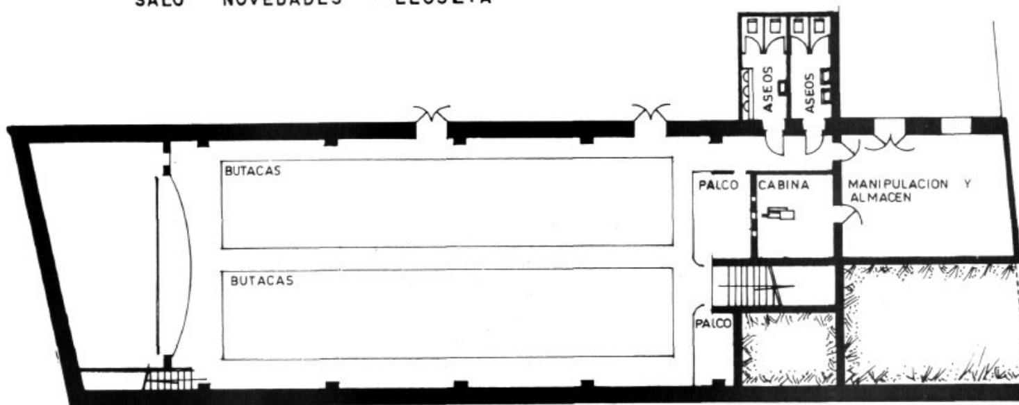
PLANTA PATI BUTACAS
