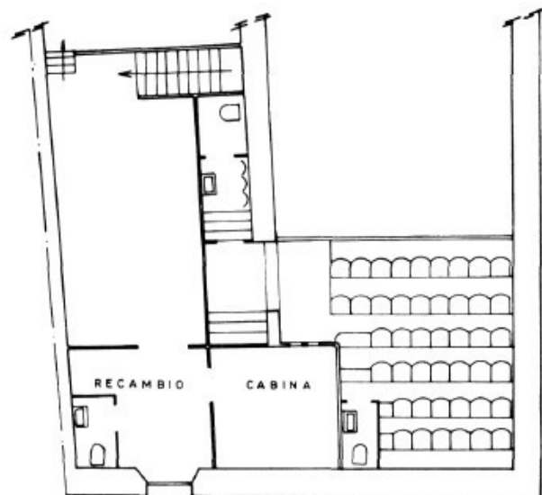
PLANTA ANFITEATRO
