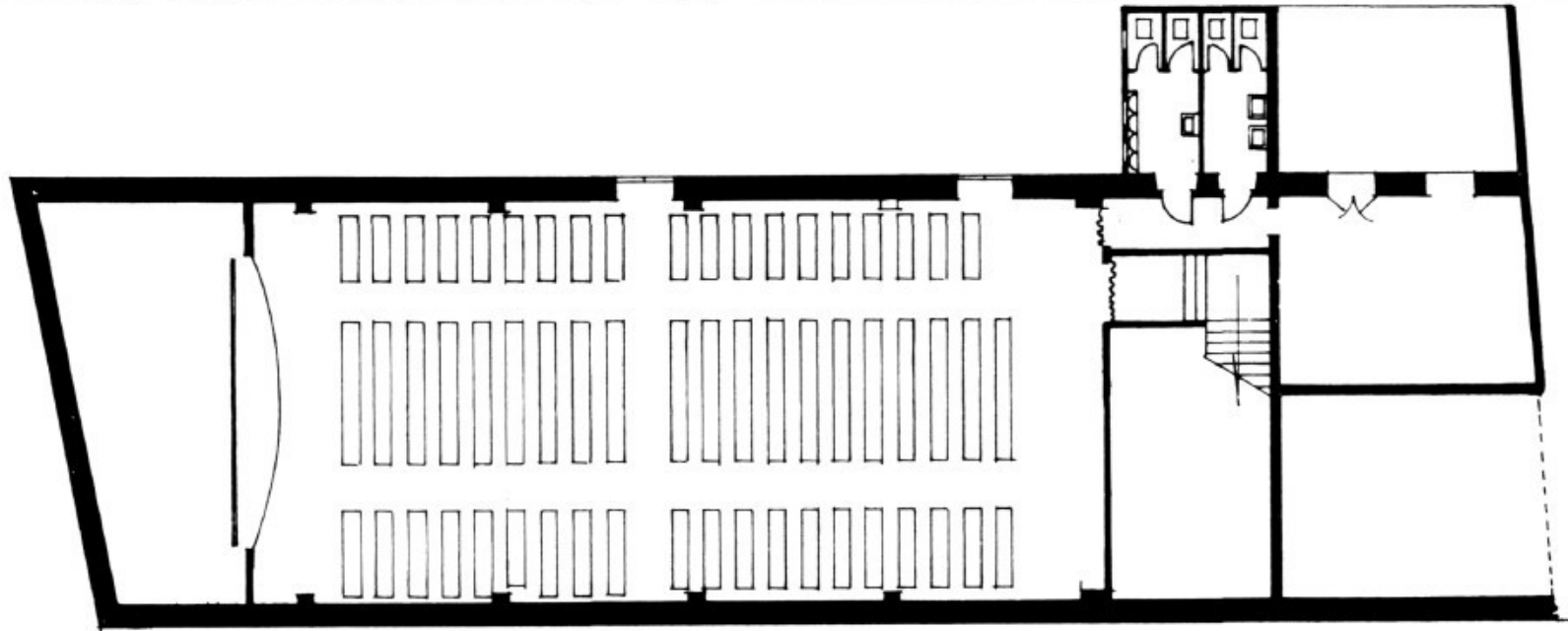
PLANTA PATIO BUTACAS
