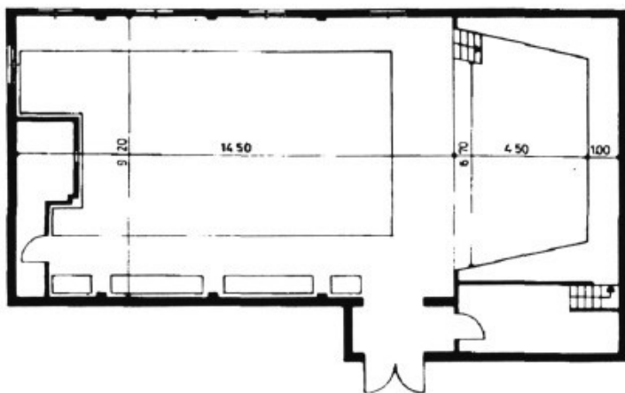
Plànol del Saló Parroquial després de la darrera reforma de 1986.
