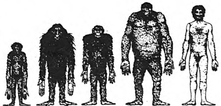
GIBÓ ORANGUTÀ XIMPANZE GORIL·LA H.SAPIENS
