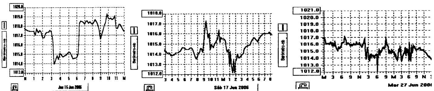
Retalls dels gràfics de la pressió atmosfèrica a S.Llorenç corresponents als moments amb més perill de risagas: font, Ca'n Xesc
