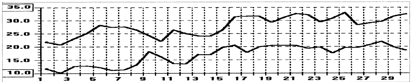
Evolució de la temperatura del mes de juny de 2006 : font Ca'n Xesc B480
