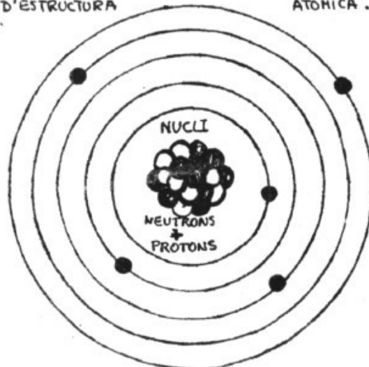
ESTRUCTURA ATÒMICA segons Rutherford
