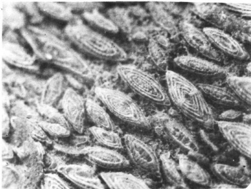
Nummulits ( Es Racó, Maria de la Salut )
