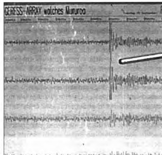
Senyes de l'explosió atòmica en un sismògraf.
