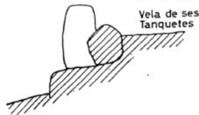
Secció
