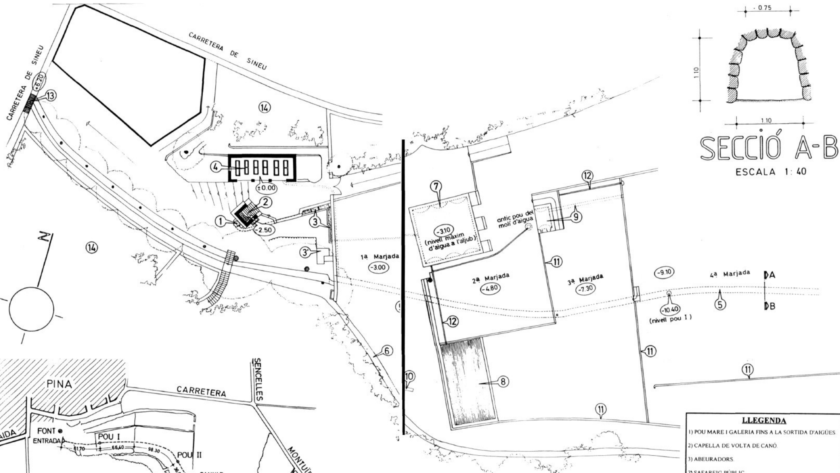
PLANTA GENERAL ESCALA 1:400
