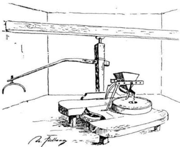
Vògit adossat a la instal·lació de les moles d'un MOLÍ DE SANG
