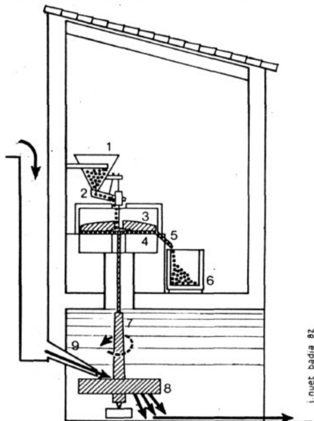
Esquema del funcionament d'un molí fariner. El recorregut del gra i de la farina, representat per punts, comença a la tremuja (1), d'on passa al canalot (2) que aconduïx el gra fins a l'ull de la mola, on cau entremig de la mola volandera (3) i de la mola sotana (4). Un cop el gra és mòlt surt pel farinal (5) i cau a la farinera (6). El recorregut de l'aigua és representat per sagetes negres. L'aigua de la bassa o del pou surt a pressió per la canal (9) i cau damunt del rodet (8), fent que volti, després s'escola pel sòl del carcavà fins a l'exterior. Les peces ratllades: el rodet (8); l'arbre (7) i la mola volandera (3) són les úniques que volten, alhora, en el molí fariner.
