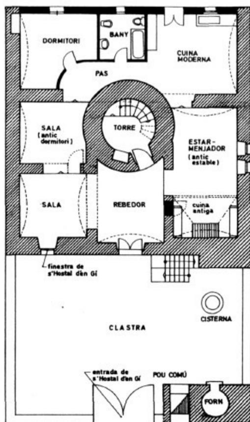
PLANTA BAIXA Escala 1:100
