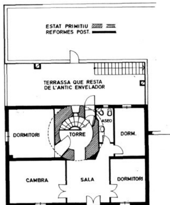
PLANTA ALTA Escala 1:200
