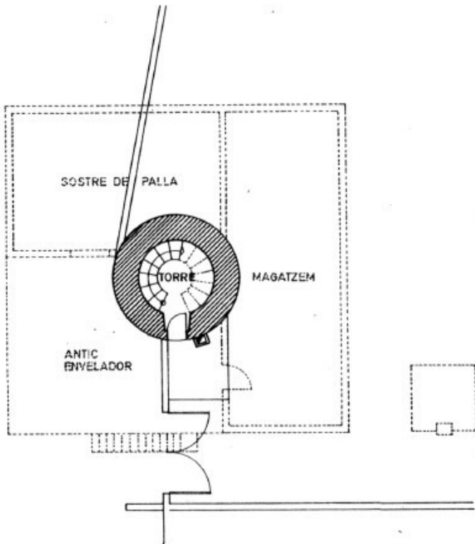
PLANTA ALTA ESCALA 1:200
