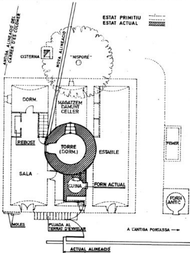
PLANTA BAIXA ESCALA 1:200
