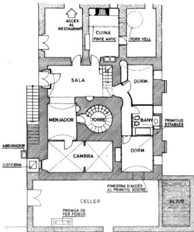
PLANTA BAIXA ESCALA 1:200
