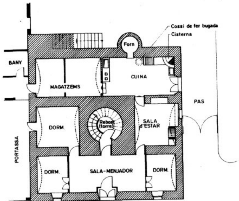
PL. BAIXA ESCALA 1:200
