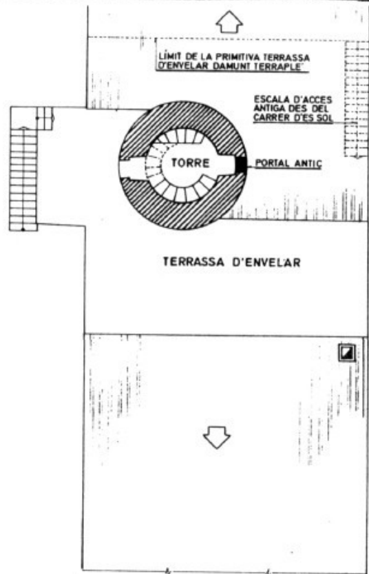
PLANTA COBERTA ESC. 1: 200
