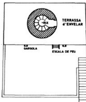
PLANTA 2a E. 1: 200
