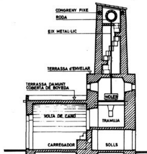
SECCIO A-B E. 1: 200
