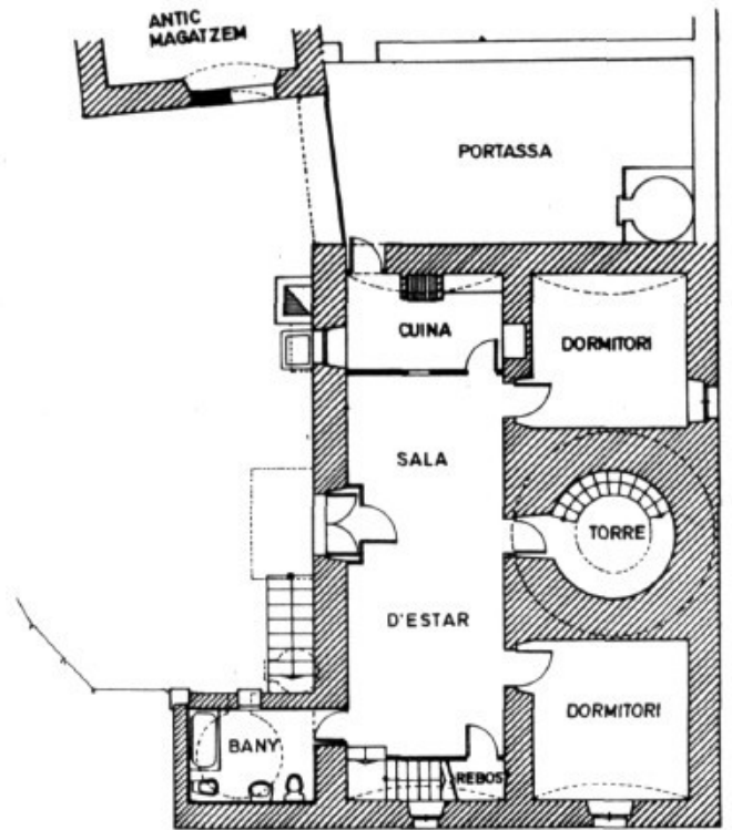
PLANTA BAIXA ESCALA 1: 200
