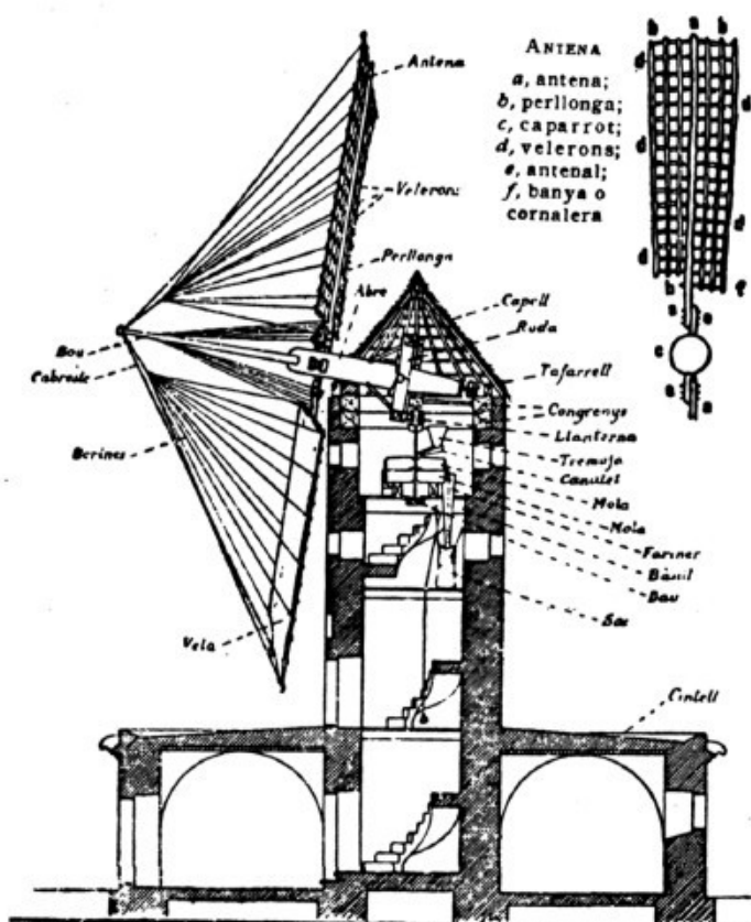
SECCIÓ VERTICAL DEL CONJUNT D'UN MOLÍ DE VENT (Dibuix de Miquel Fullana)
